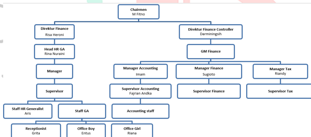
Gambar 2.1 Struktur Organisasi
