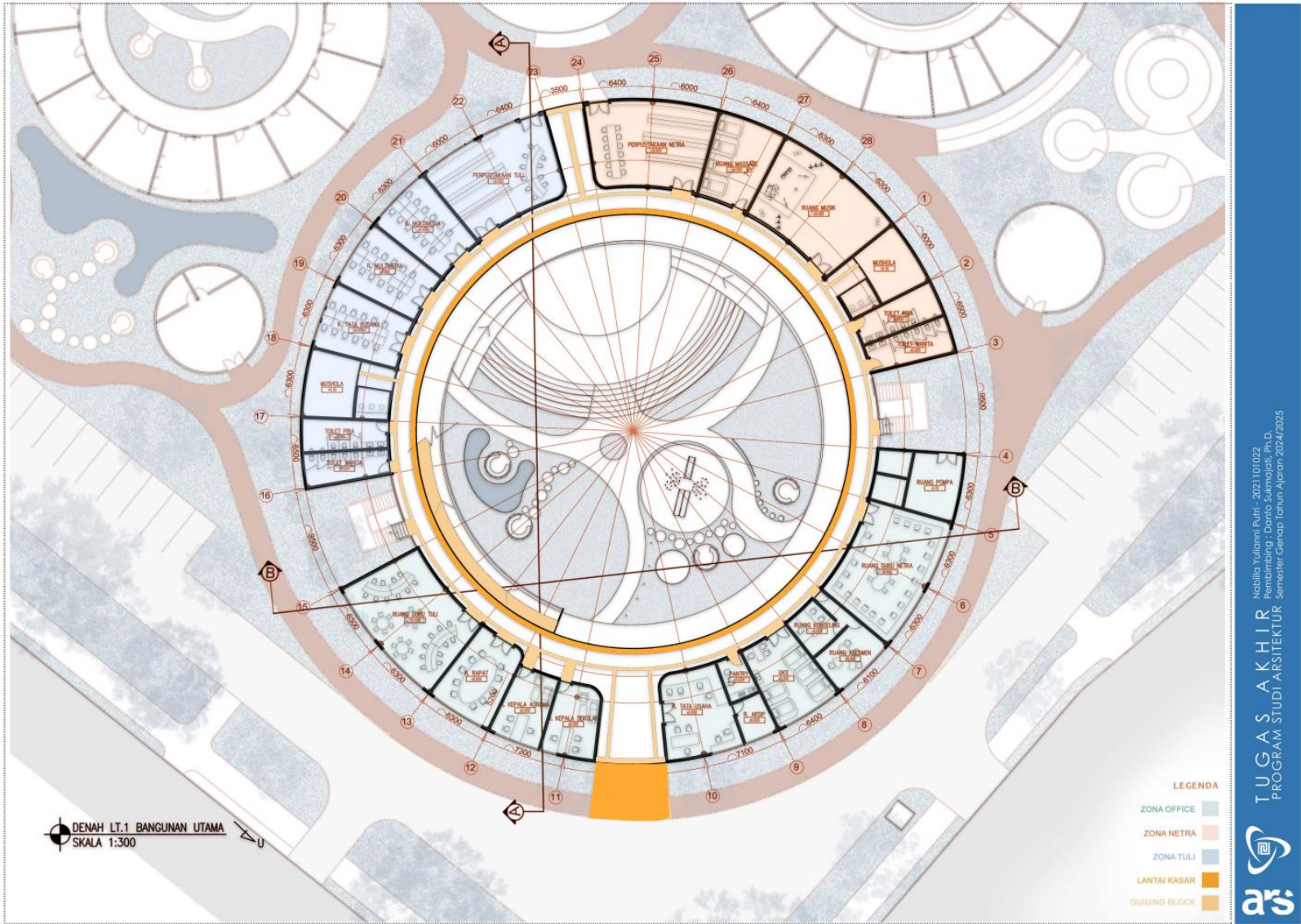
Lampiran 7. Denah Lt.1 Bangunan Utama
