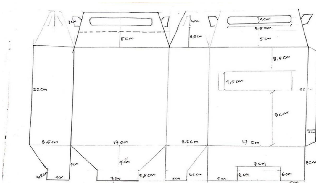
Gambar 3 : Gambar Potongan
