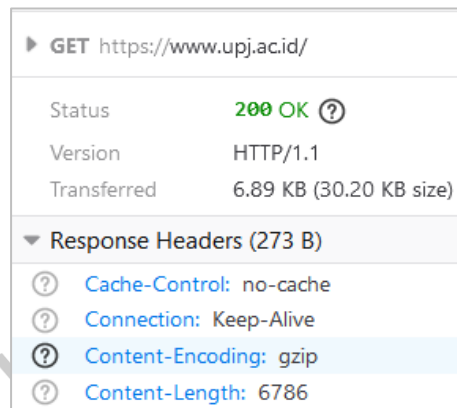
Gambar 3. 15 Cek status kompresi GZip Sumber: Dokumentasi praktikan
