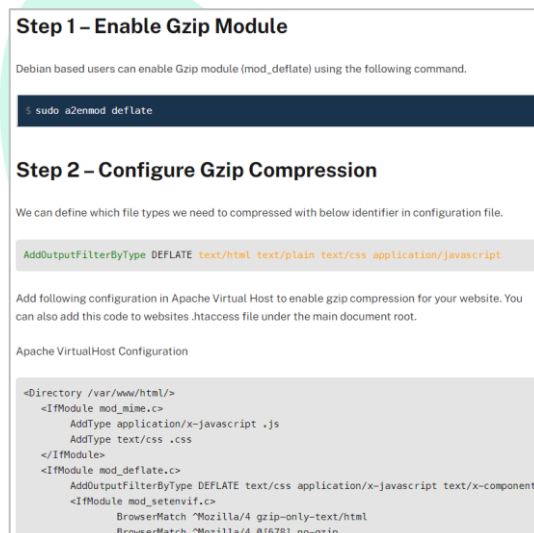
Gambar 3. 14 Konfigurasi GZip Sumber: Dokumentasi praktikan
