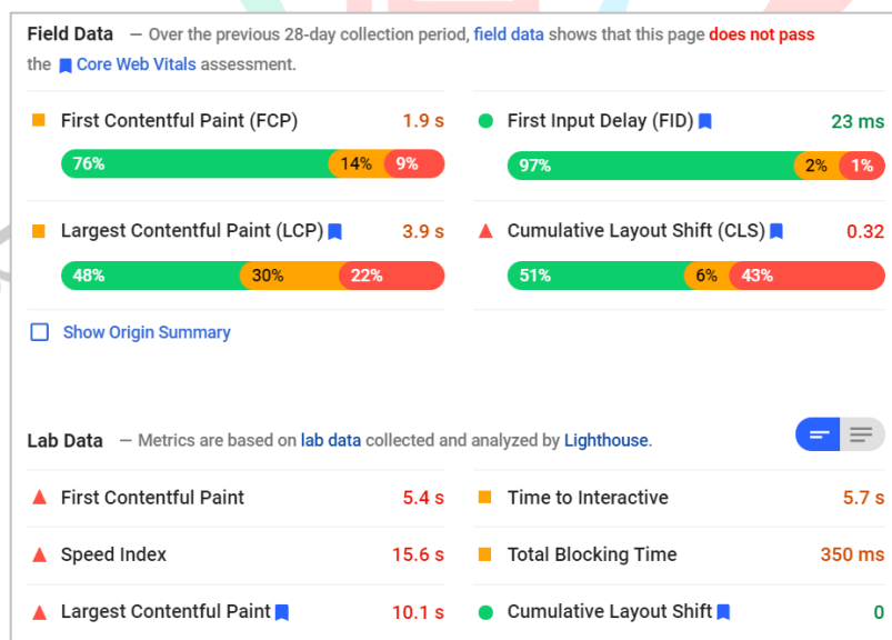
Gambar 3. 5 Field Data dan Lab Data
