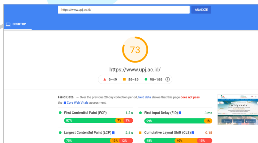
Gambar 3. 4 Skor PageSpeed Insights versi desktop Sumber: Dokumentasi praktikan
