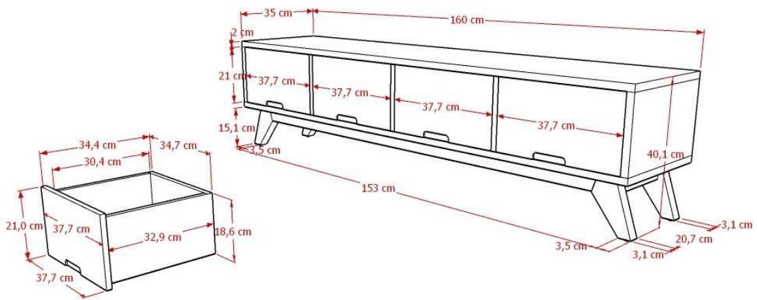
Lampiran 2.11. Membuat Dimensi Ukuran Produk Uwitan
