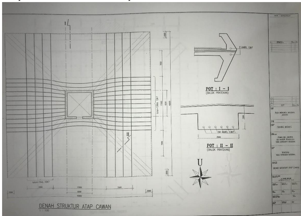
Lampiran 3 Denah Struktur Atap Cawan
