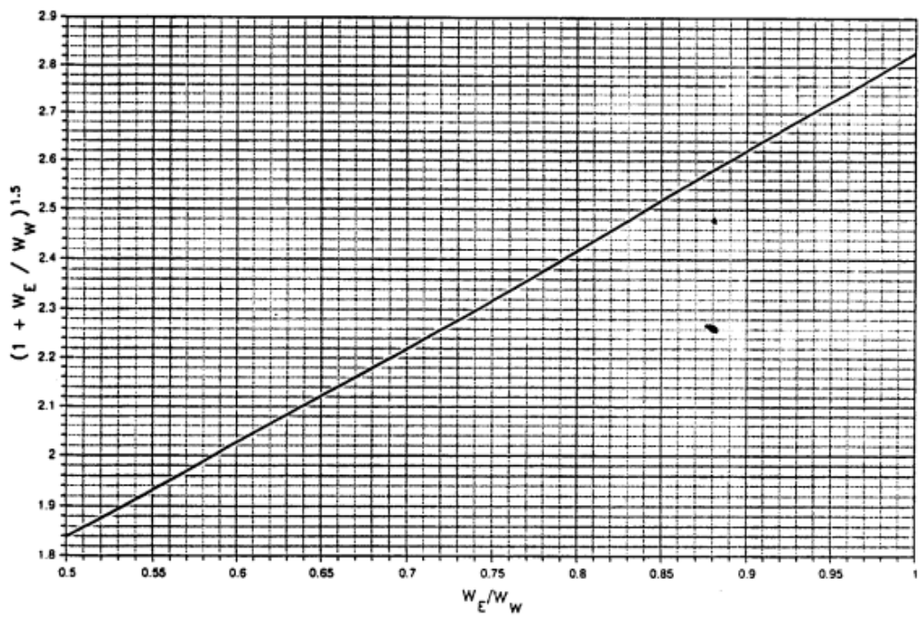
Lampiran 2 Nilai (1 + W_E/W_w)^{1.5} Terhadap W_E/W_w
