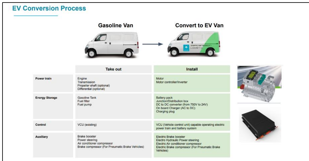
Gambar 2. 3 Proses konversi kendaraan mesin bensin menjadi listrik
