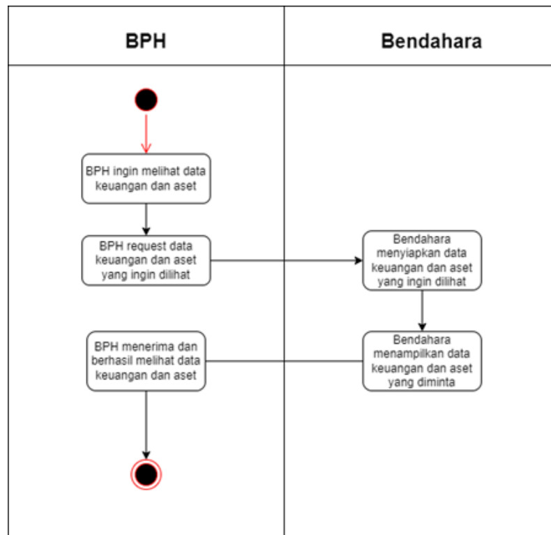
Gambar 3.7. Diagram activity melihat data keuangan dan aset
