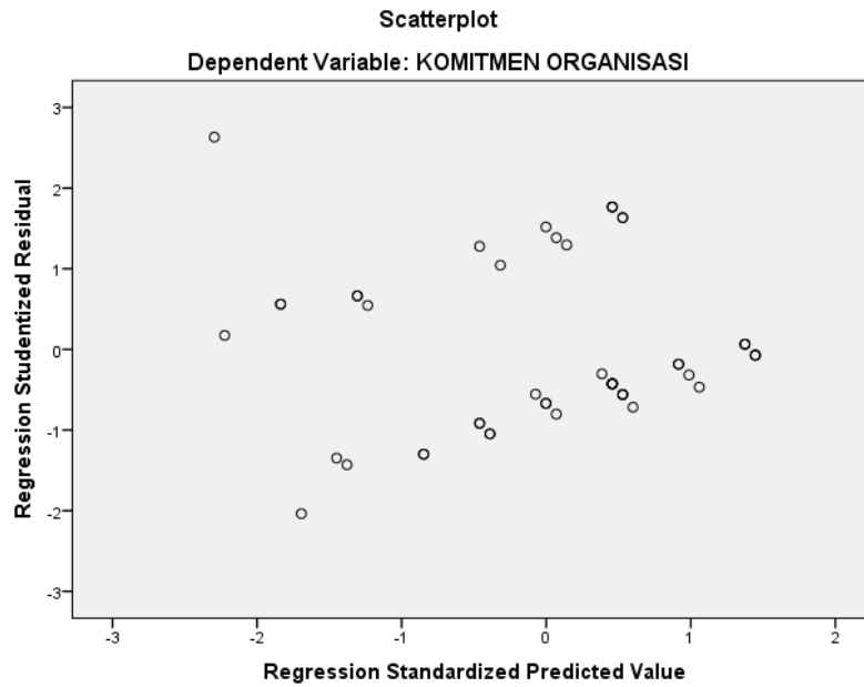
Gambar 4.1 Hasil Uji Heterokedasitas
