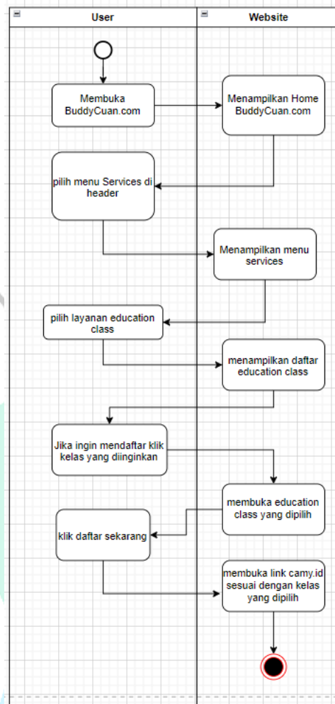
Gambar 3.6 Act Diagram Melihat dan Mendaftar Education Class
