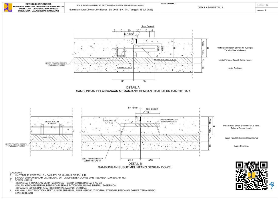
Lampiran 2. 5 Denah Sambungan, Spesifikasi, dan Potongan Rigid Pavement yang Digunakan Pada Proyek Tol Serpong-Balaraja Seksi 1B
