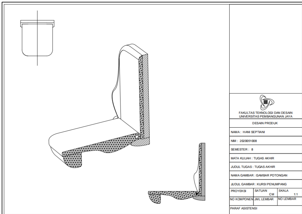
Lampiran 8. Gambar Potongan Kursi Penumpang (dok.pribadi)
