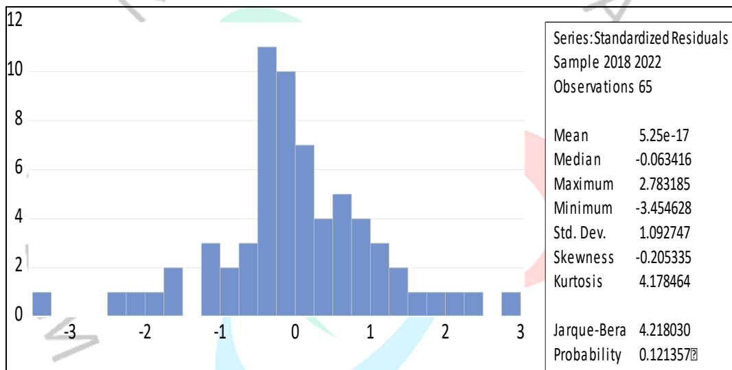
Gambar Uji Normalitas
